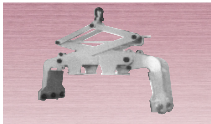
古紙プレス圧縮成形品吊具
