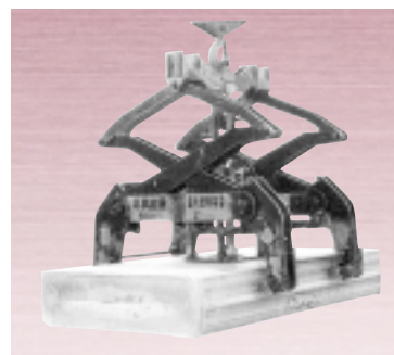
自動着脱型 アルミスラブ吊具
