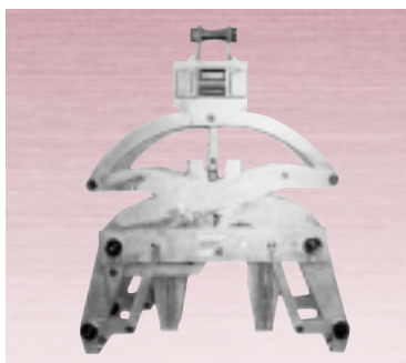
自動着脱型 スラブ吊具
