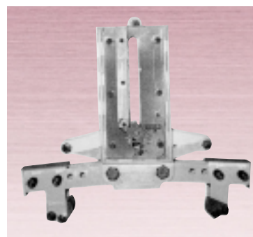
自動着脱型 爪ポイント式 インゴット吊具
