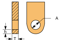
ホイスト取付部フック寸法
