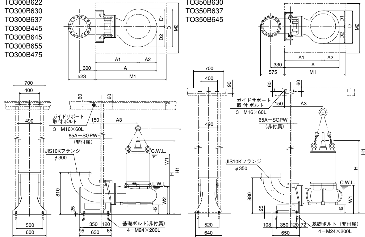
寸法表 単位: mm
