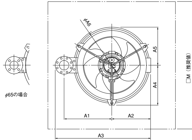
■外形据付寸法図 (例) 単位: mm
