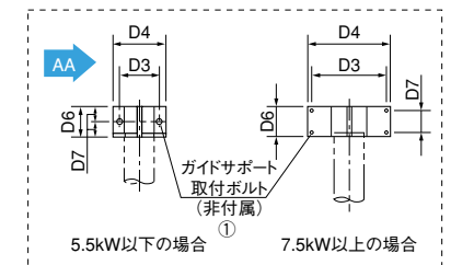
ガイドサポート (非付属) 部
