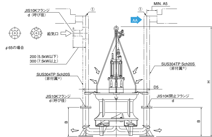
寸法表
